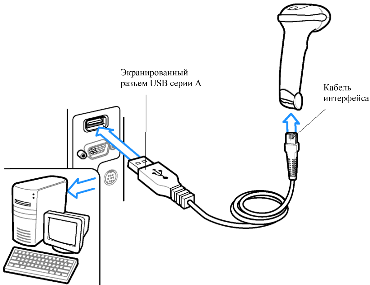
Рисунок 5-1 Подключение к USB
