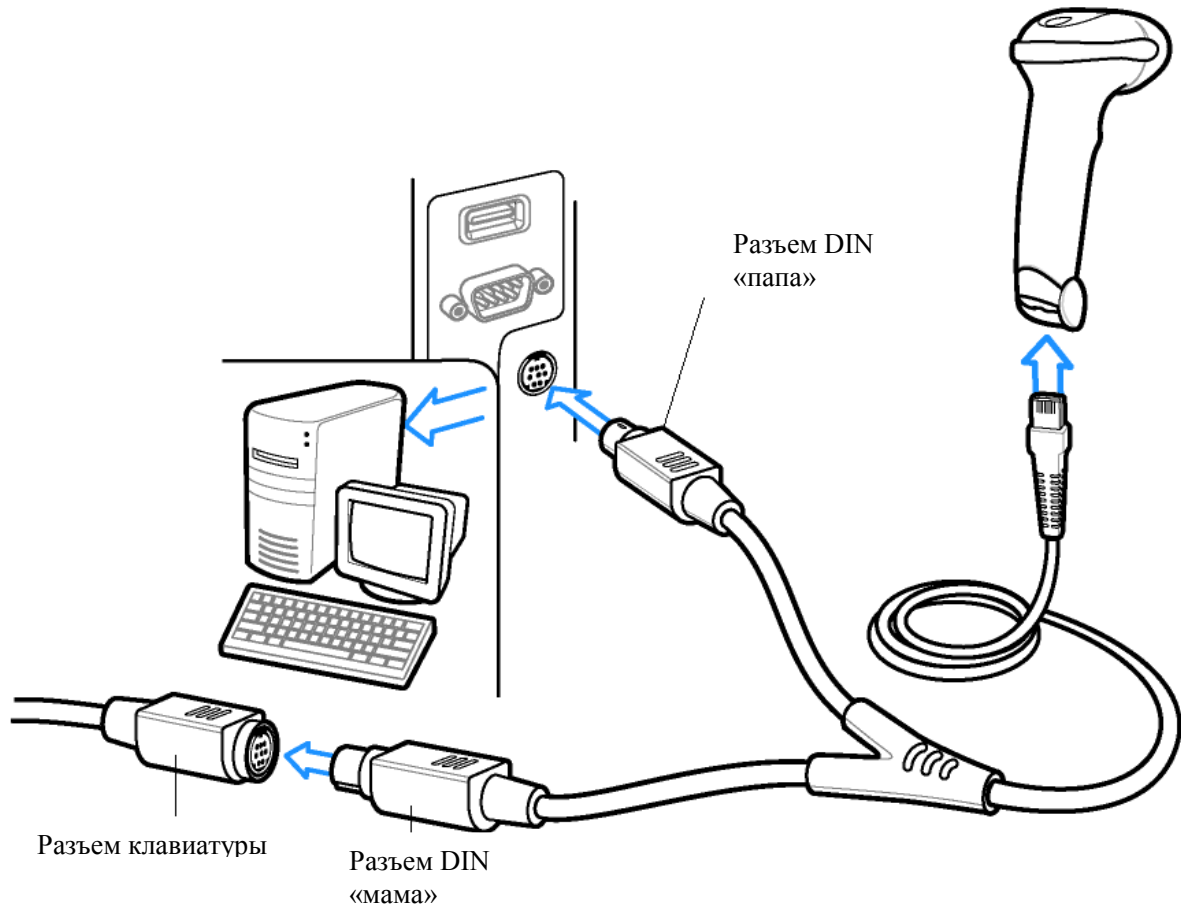
Рисунок 8-1 Подключение Keyboard Wedge с Y-образным кабелем
