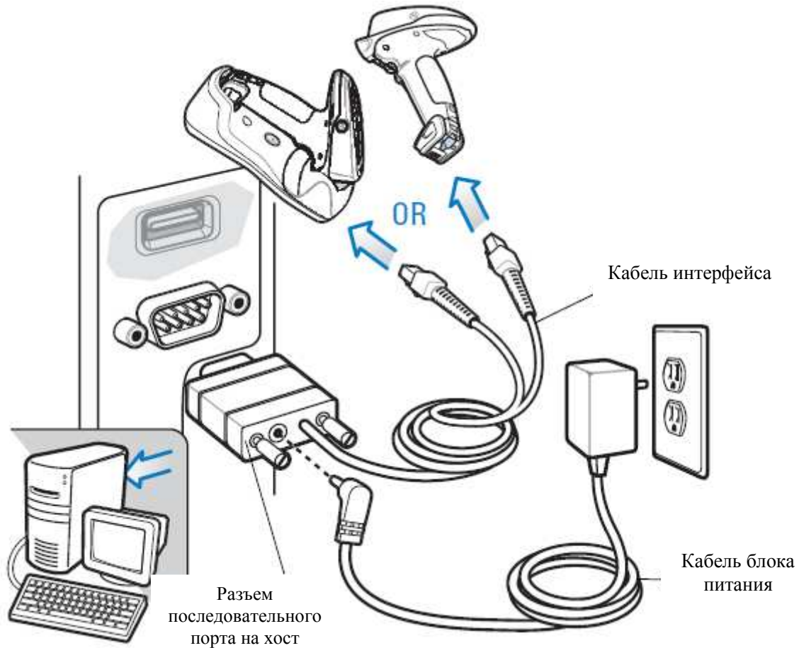
Рисунок 8-1 Прямое подключение RS-232
