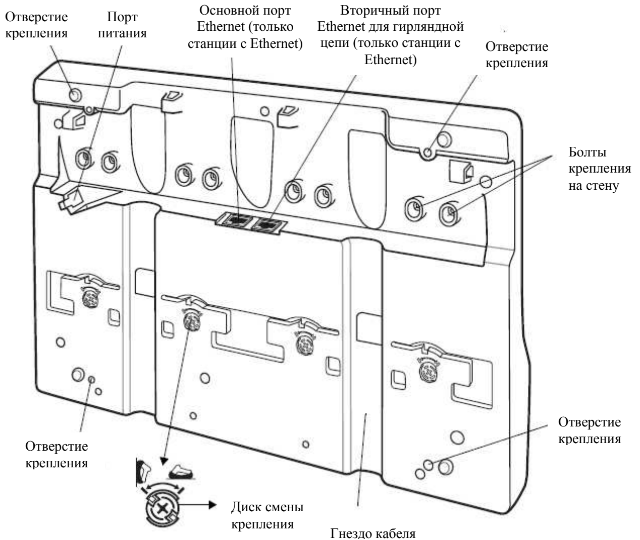
Рисунок 1-6 Базовая станция с 4 гнездами – вид сзади
