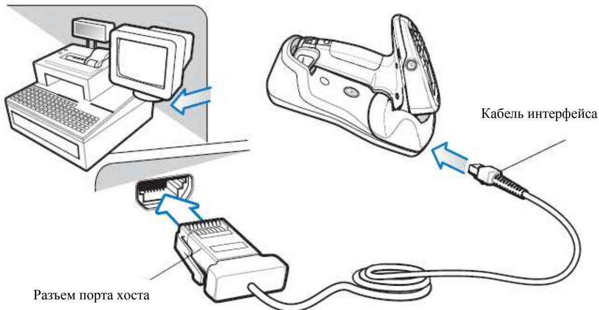
Рисунок 10-1 Прямое подключение IBM
