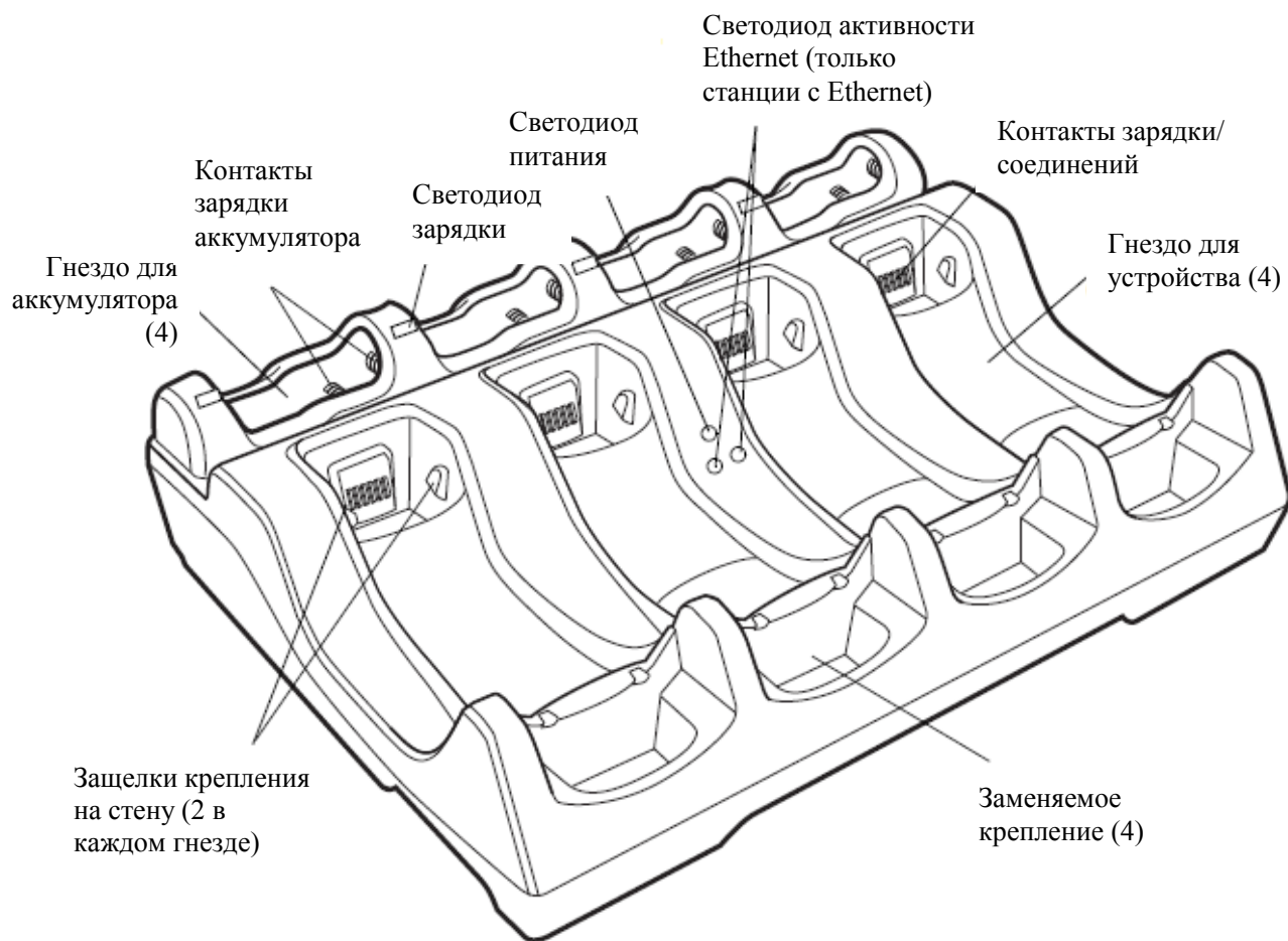
Рисунок 1-5 Базовая станция с 4 гнездами – вид спереди
