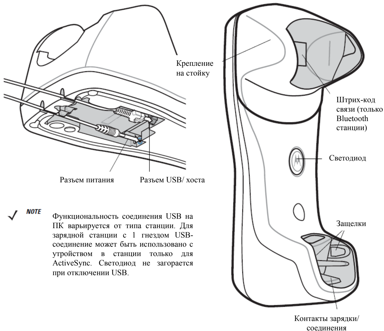
Рисунок 1-2 Базовая станция с 1 гнездом – соединения/ штрих-код связи
