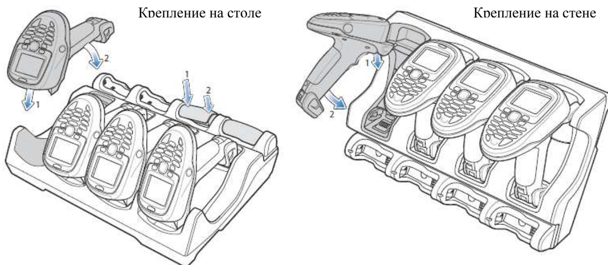
Рисунок 13-1 Вставка устройства в базовые станции на столе и на стене
