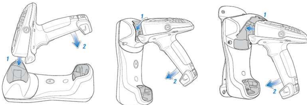
Рисунок 1-9 Вставка устройства в базовые станции с 1 гнездом
