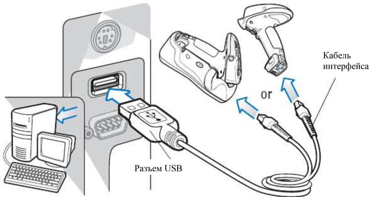
Рисунок 9-1 Подключение к USB
