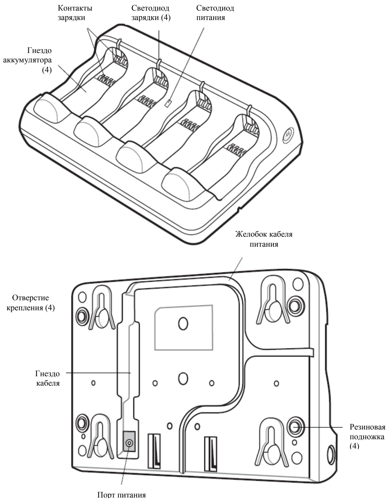
Рисунок 1-7 Зарядное устройство запасных аккумуляторов с 4 гнездами
